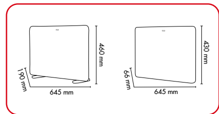
Dimensioni Dimensions
