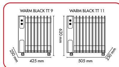
Dimensioni Dimensions
