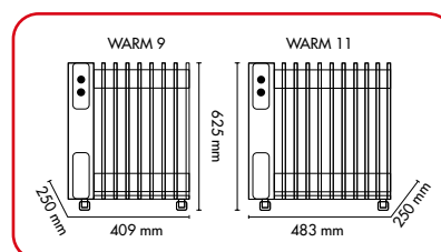
Dimensioni Dimensions
