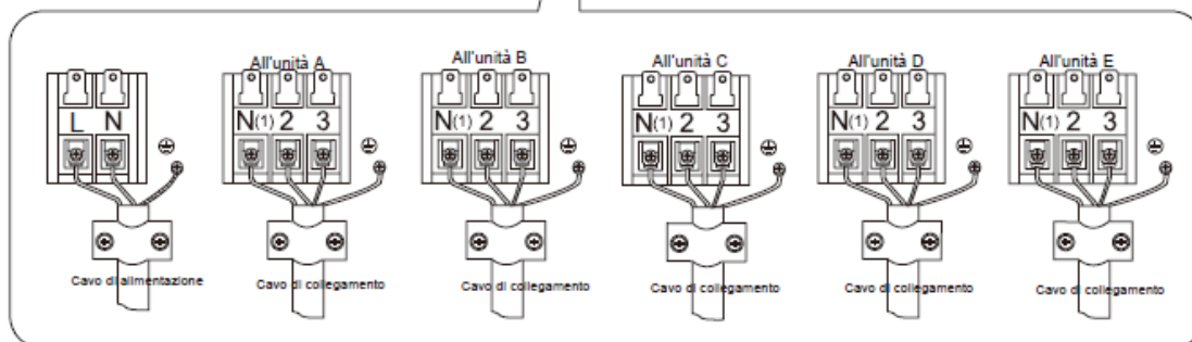
All'alimentazione elettrica
