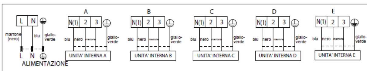
All'alimentazione elettrica
